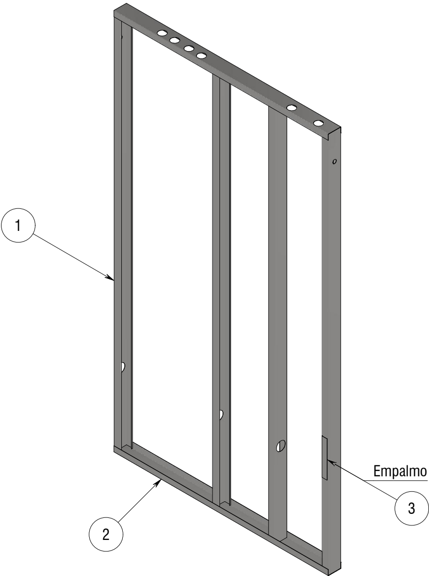
ISOMÉTRICO ( 1 : 15 )
