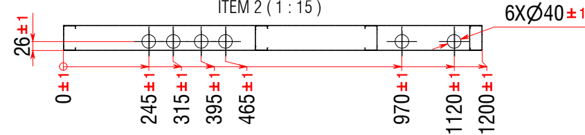
ITEM 2 ( 1 : 15 )
