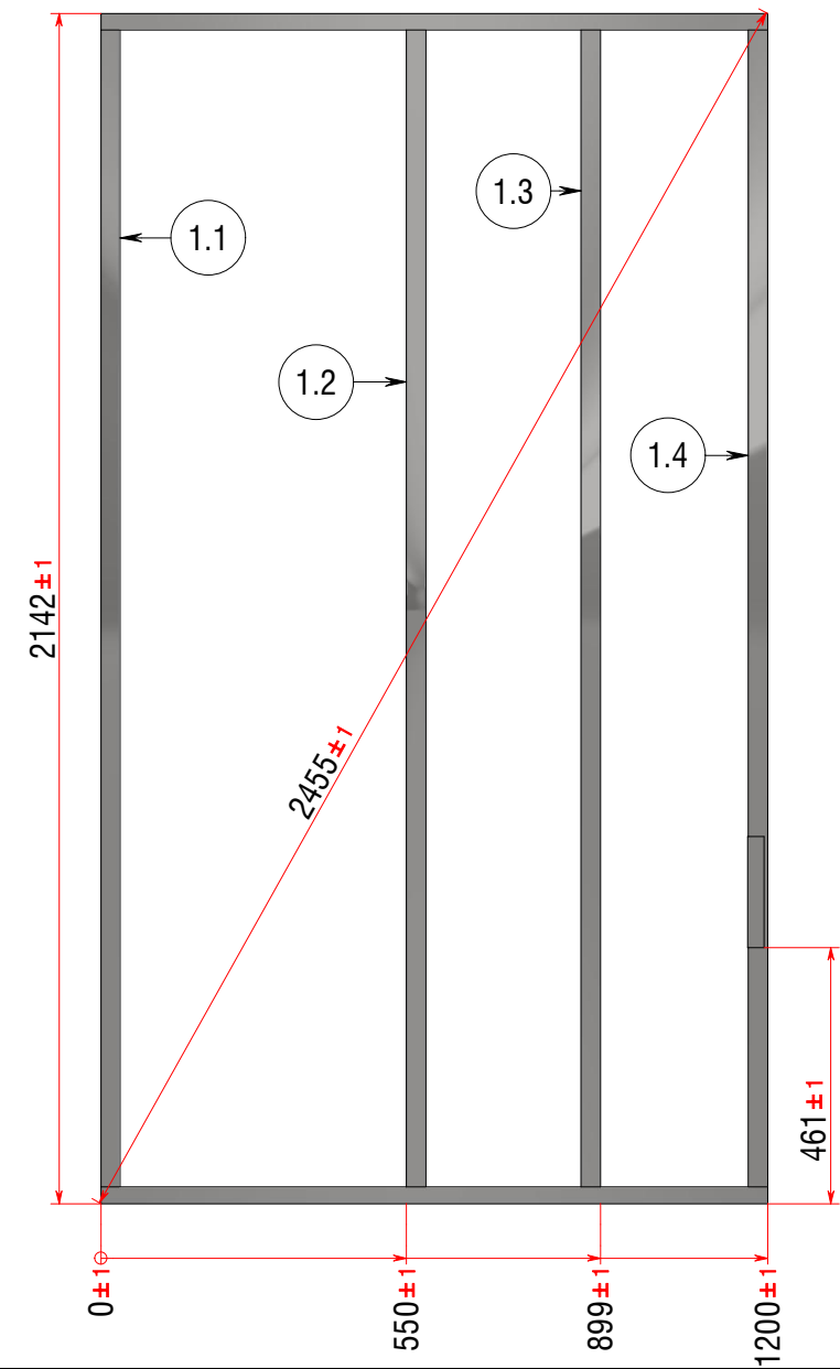
ITEM 2 ( 1 : 15 )
